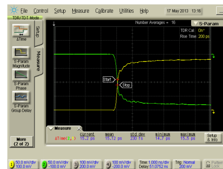
Skew
